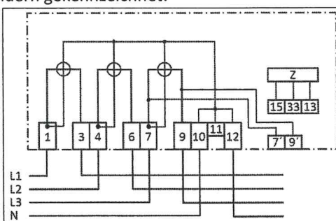
Abb. 3: Schaltung 4102 (Doppeltarif)
