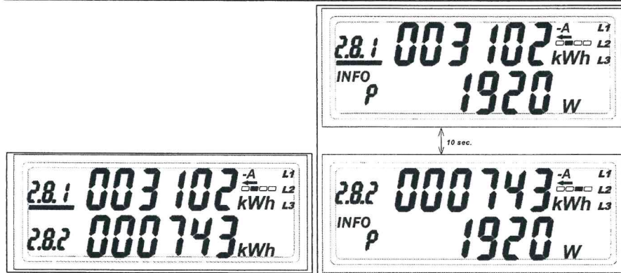
Abb. 12: Doppeltarif-Lieferzähler ohne (links) und mit (rechts) Leistungsanzeige
