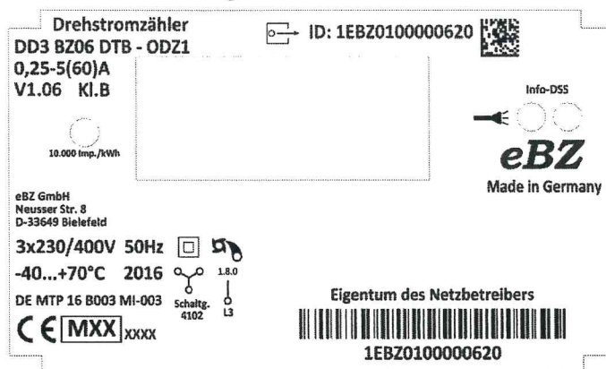
Abb. 4: Leistungsschild des DD3 (Beispiel)
